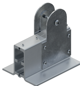
Base autoportante EN 13374
