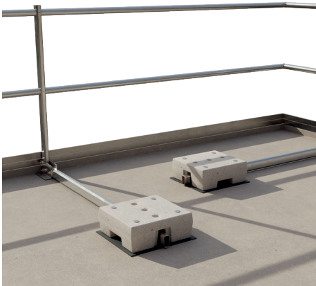
Ausführung 2 - mit Brüstung \geq 5 cm < 15 cm
