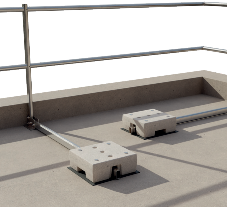
Ausführung 1 - mit Brüstung \geq 15 cm
