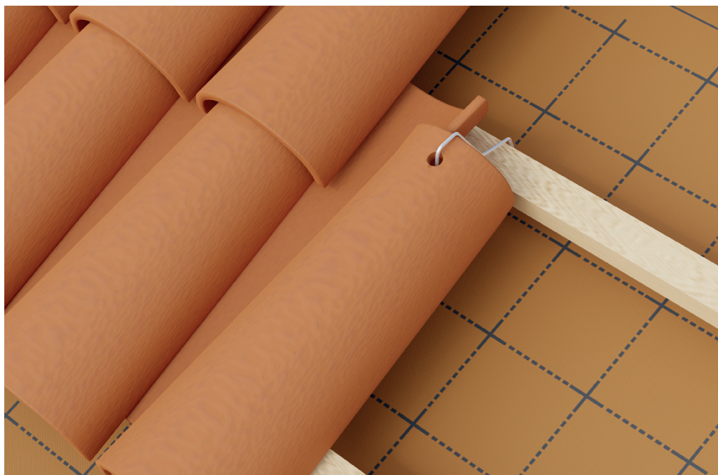
Crochet contrevent pour tuile perforée
