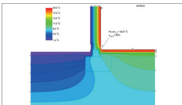
ISOTHERMISCH GEPRÜFT
