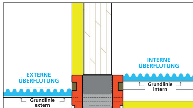
KEINE WASSERSTAGNATION
