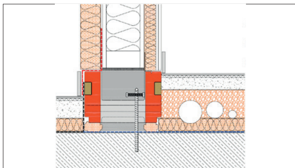
ANWENDUNGSSCHEMA
